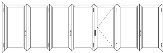
finestra 7 ante scorrevoli a libro (4+3)* 7 panel folding window (4+3)
